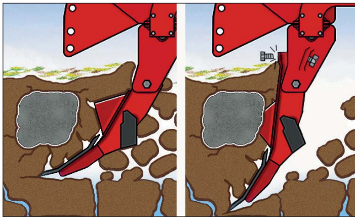
V základním provedení jsou slupice jištěné střížnou pojistkou
